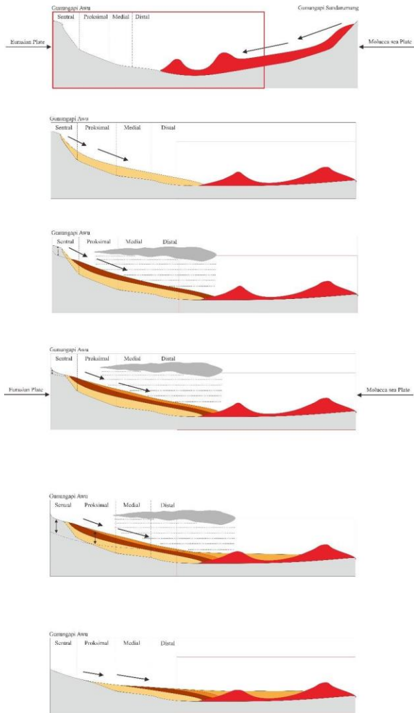
Gambar 16. Permodelan Sejarah Geologi
